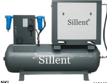
HAVA KURUTUCU
